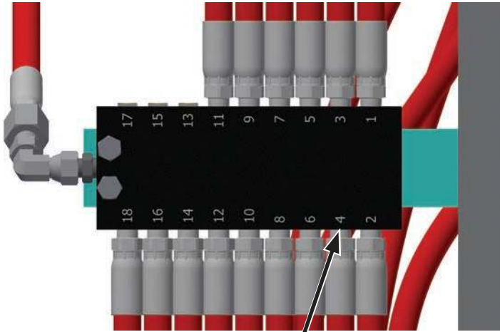
Detalle de la válvula divisora de engrase
